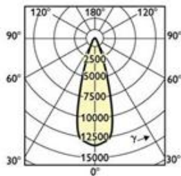
CDM-R 70W / PAR30L / 30D
