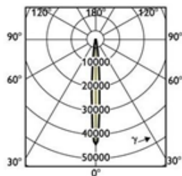
CDM-R 35W / PAR30L / 10D
