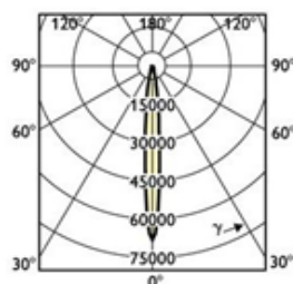
CDM-R 70W / PAR30L / 10D
