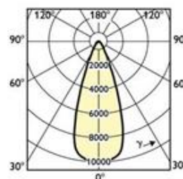
CDM-R 70W / PAR30L / 40D
