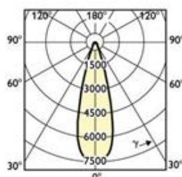
CDM-R 35W / PAR30L / 30D
